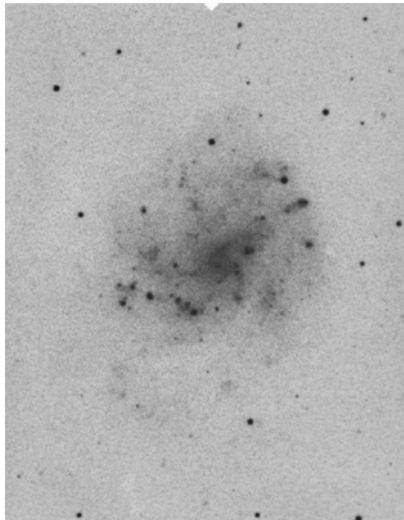
3 MCG-1-57-16 (G) p. 166
