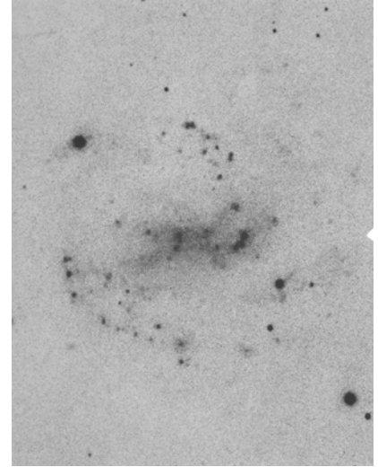
2 UGC 10310 (P) p. 246
